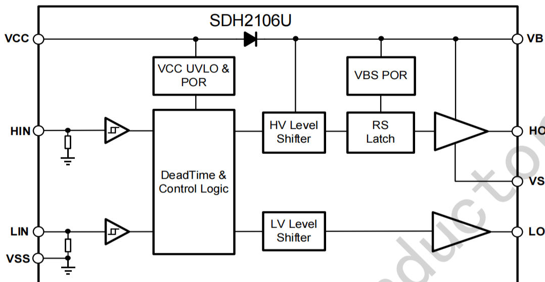
图 7-1 SDH2106U的功能框图
