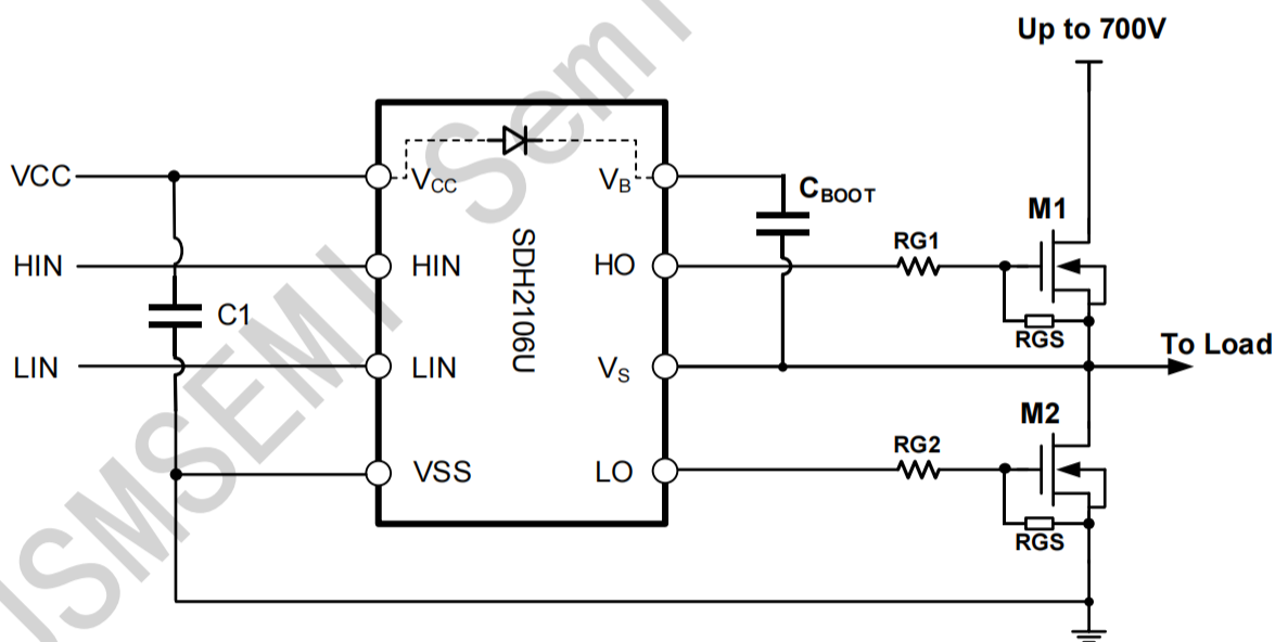
图 7-2 SDH2106U典型应用电路图
