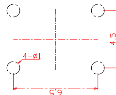
PCB. 焊接图
