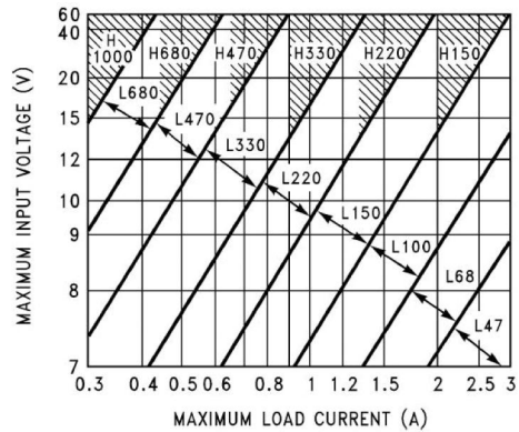
LM2576-5.0
