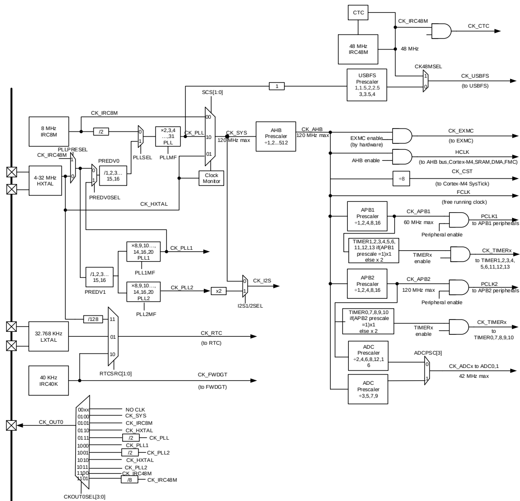
Figure 2-7. GD32C103xx clock tree
