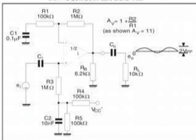
图3. 交流耦合正向放大器
