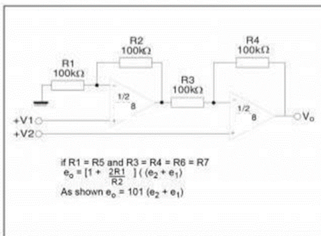
图5. 高输入阻抗,直流差分放大器
