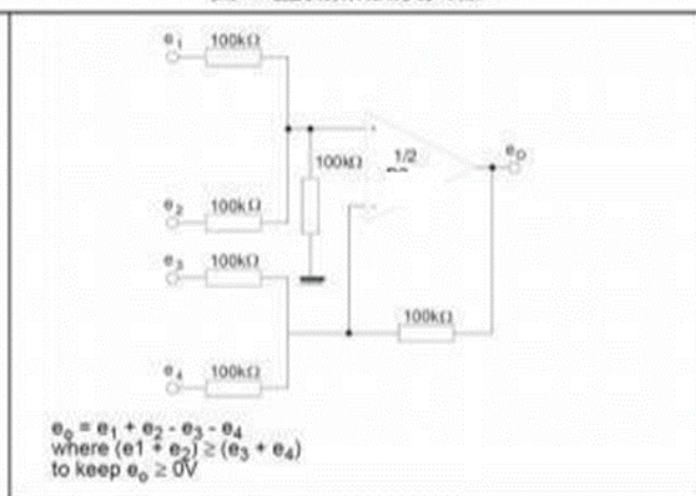
图4. 直流加法放大器
