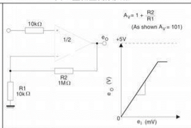
图2. 直流正向放大器
