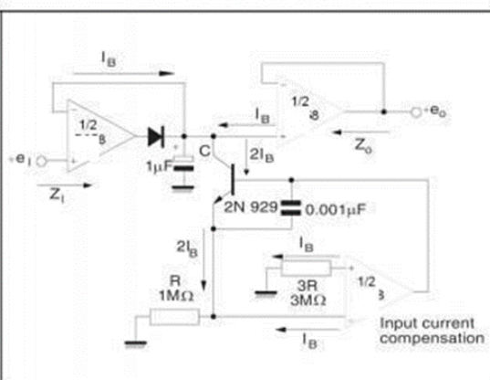
图8. 低漂移峰值检波器
