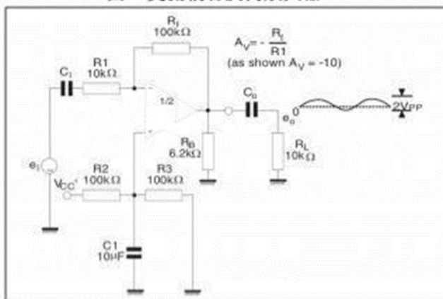
图1. 交流耦合反向放大器
