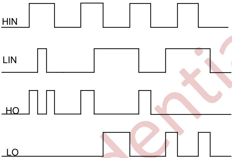
图 9-1 NSG3023 输入输出时序波形
