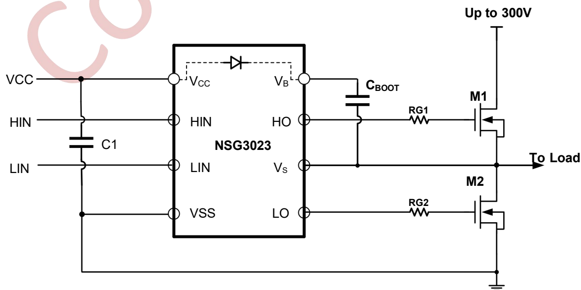
图 10-2 NSG3023 典型应用电路图
