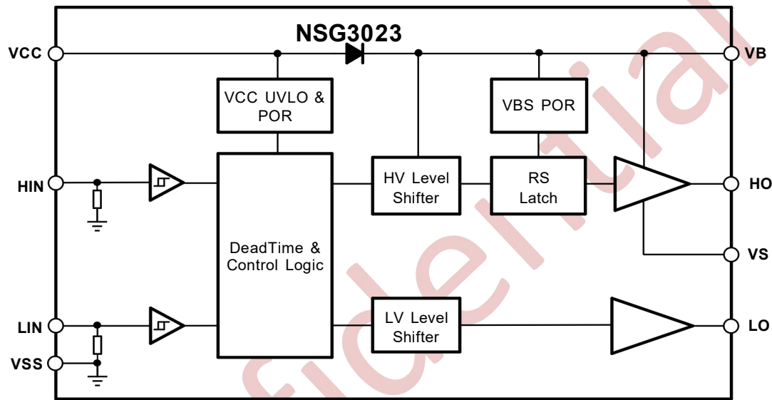
图 10-1 NSG3023 的功能框图
