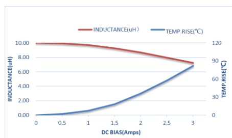
ZETC303015D100MBT-LF
