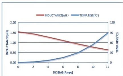
ZETC303015D1R5MBT-LF
