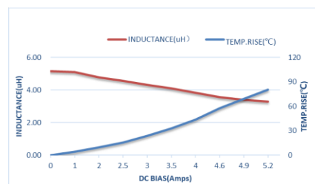
ZETC303015D4R7MBT-LF
