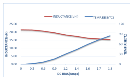
ZETC303015D220MBT-LF
