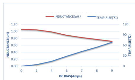
ZETC303015D1R0MBT-LF
