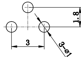
PCB线路板安装图(±0.1)
