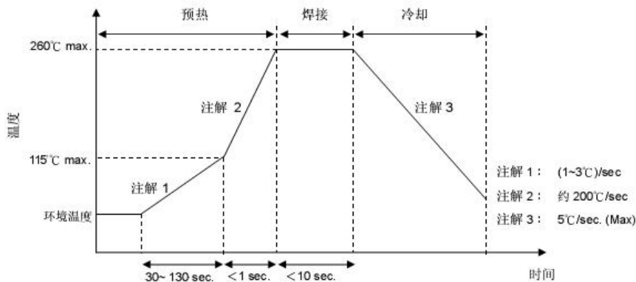
波峰焊曲线
