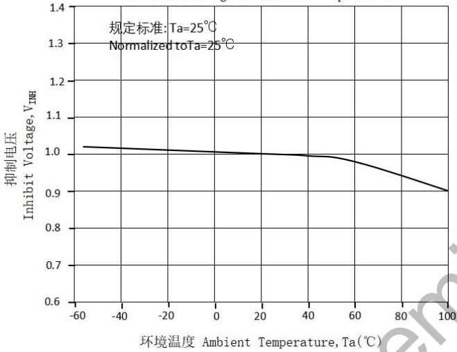
图9. 抑制电压与环境温度 Inhibit Voltage vs Ambient Temperature
