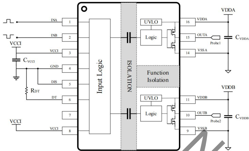
图 28 死区时间的测试电路
