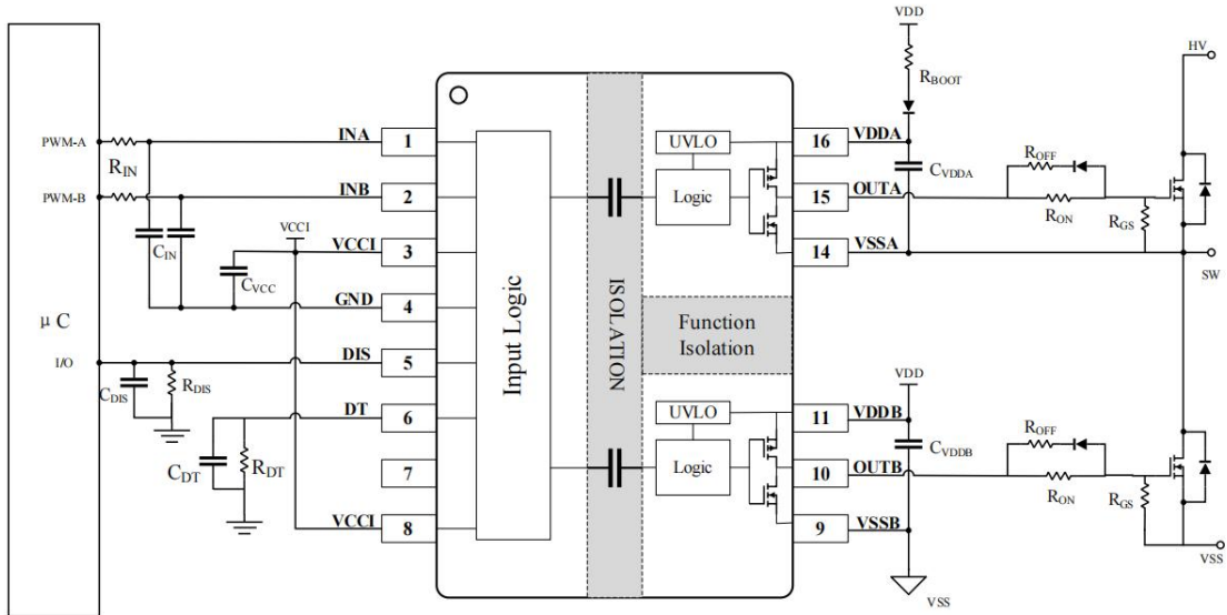
图 1 典型应用图
