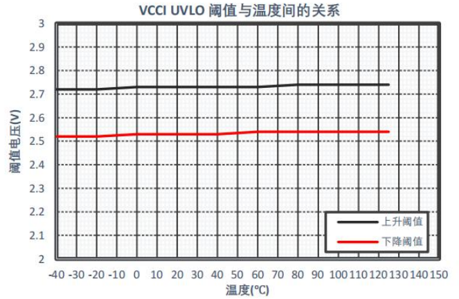
图 14 VCCI UVLO 阈值与温度间的关系
