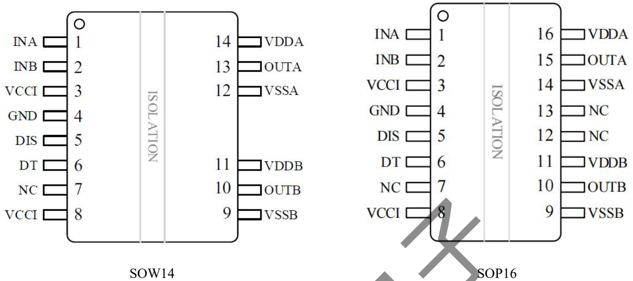
图2 引脚排列图（顶视图）
