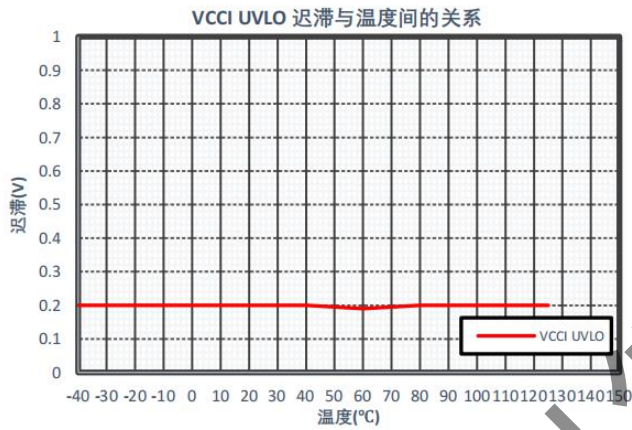
图 15 VCCI UVLO 迟滞与温度间的关系
