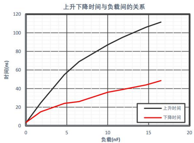
图6 上升下降时间与负载间的关系
