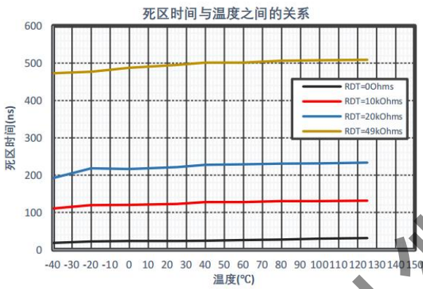
图 21 死区时间与温度间的关系
