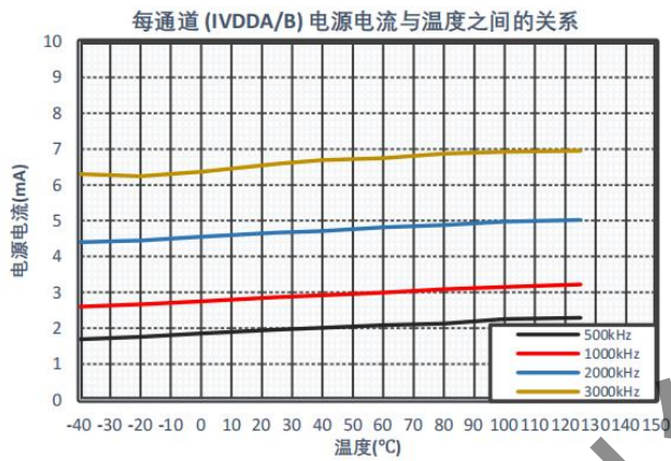
图9 动态电源电流(IVDDA/B)与温度之间的关系
