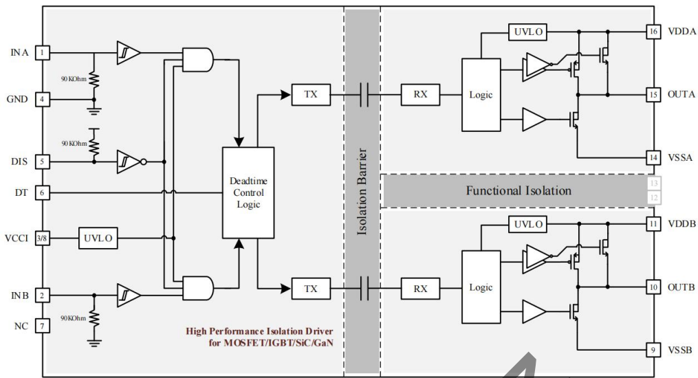
图 33 功能框图
