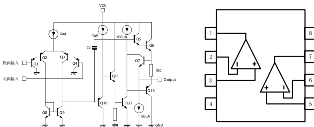
LM2904的内部原理图
