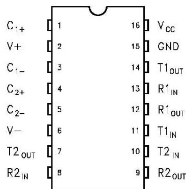
DIP-16/SOP-16/TSSOP-16
