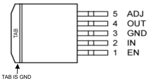
TO-263-5
