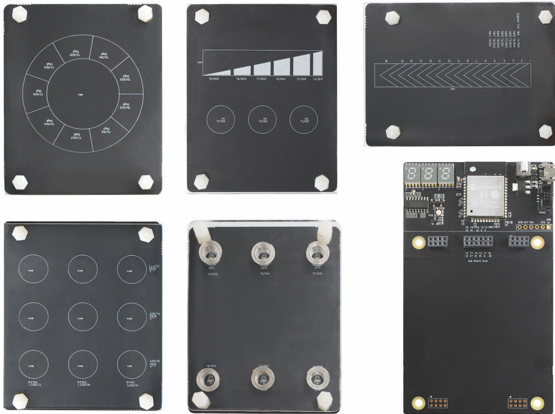
Fig. 1: ESP32-Sense-Kit
