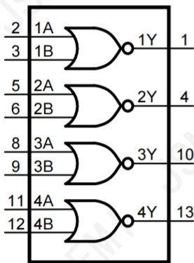
图 1 逻辑符号
