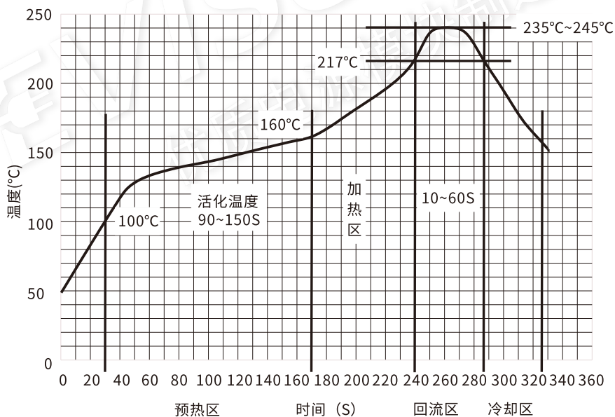
SMD 封装产品过回流焊参考曲线
