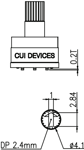
ACTUATOR
