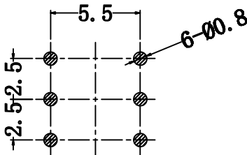
PCB参考图
