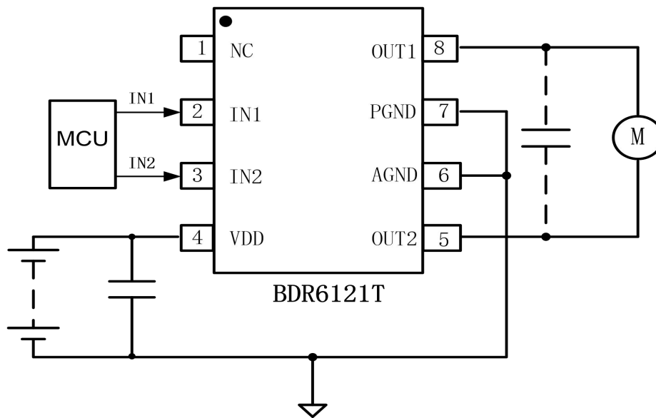
典型应用电路原理示意图
