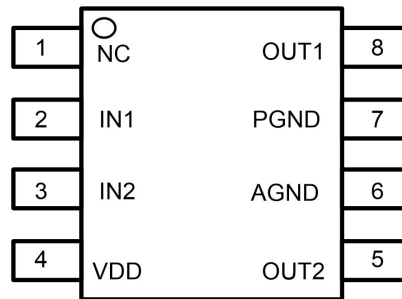
BDR6118-SOP8
