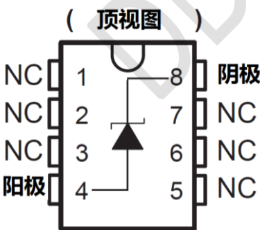
图 4 SOP8 管脚图
