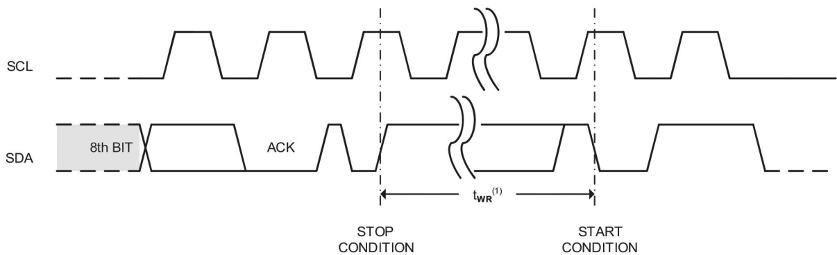
图2 总线时序
