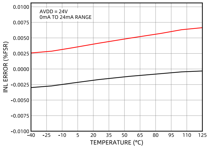
图 14 INL 的温度特性 (内部电阻)
