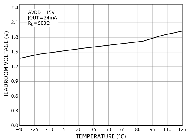
图 26 净空电压的温度特性
