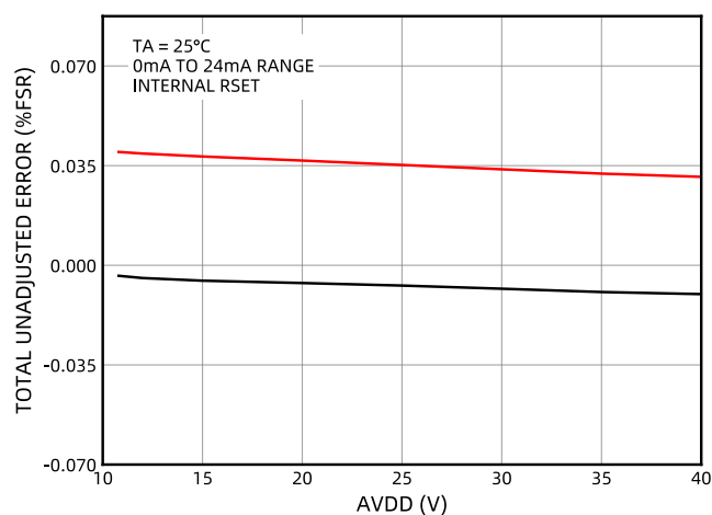
图 25 TUE vs AVDD (内部电阻)
