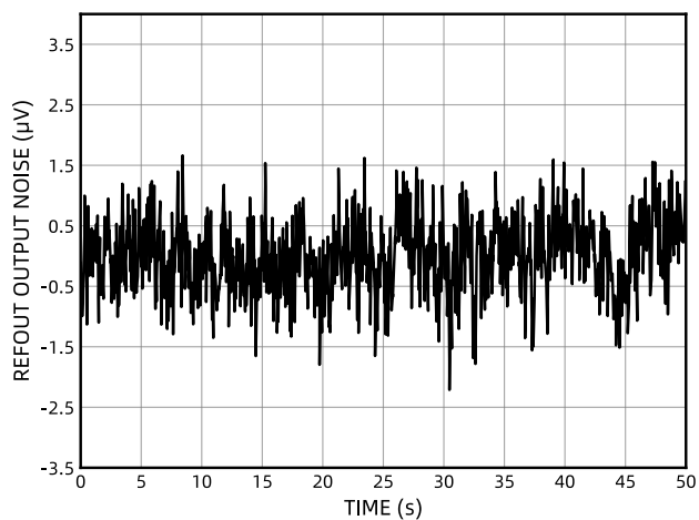
图 8 REFOUT 输出噪声 (0.1Hz~10Hz)
