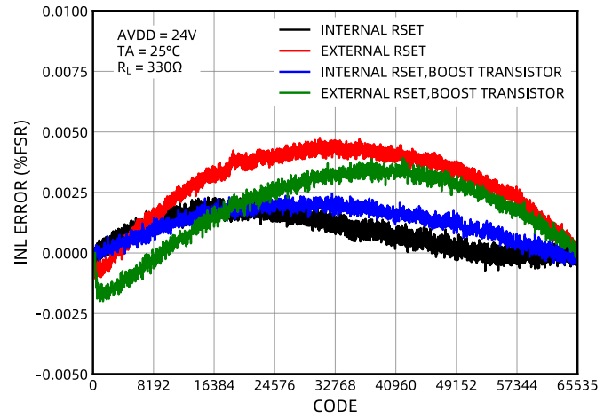
图 11 INL vs DAC 码值
