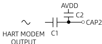
图 36 HART 信号耦合
