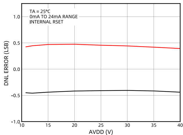
图 23 DNL vs AVDD (内部电阻)
