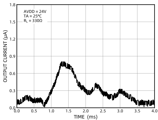
图 27 上电输出电流随时间的变化
