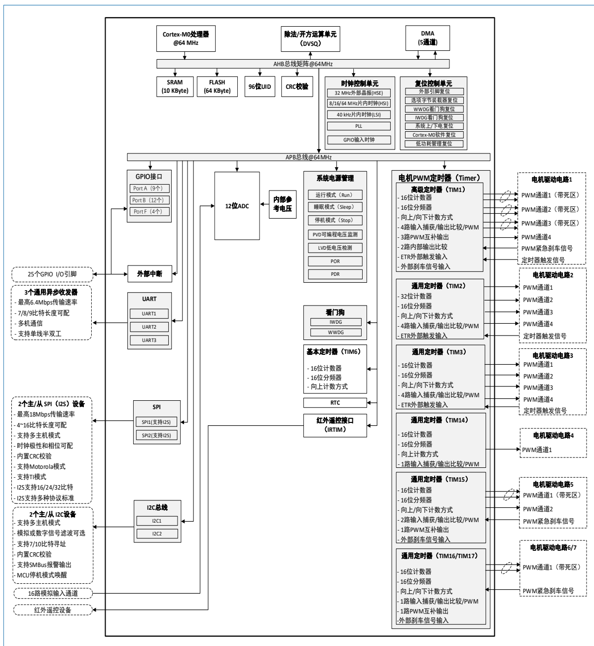
图 3-1 HK32C005K8T7 功能框图
