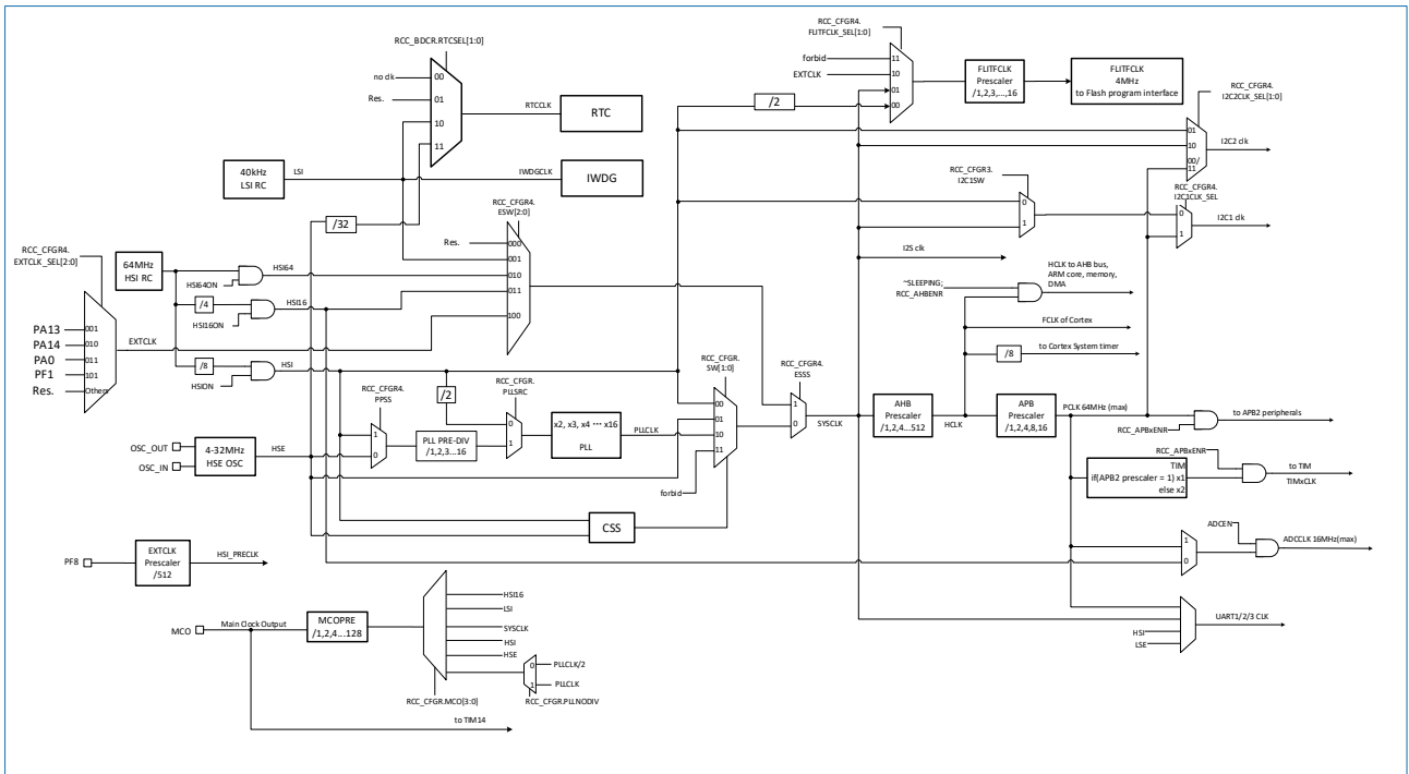
图 3-4 时钟树
