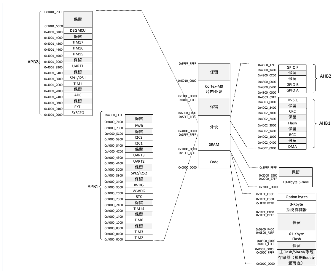
图 3-2 HK32C005 存储器映射
