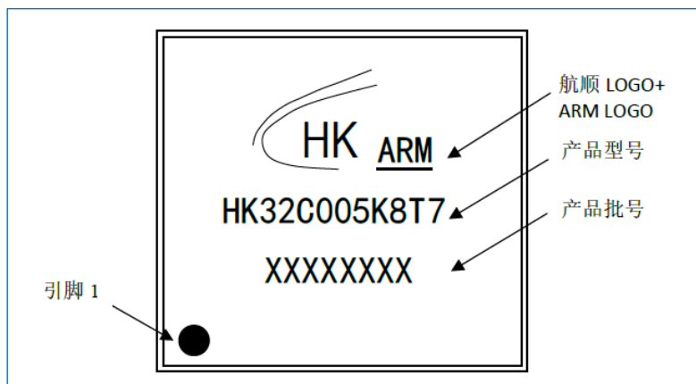
图 7-2 LQFP32 丝印示例
