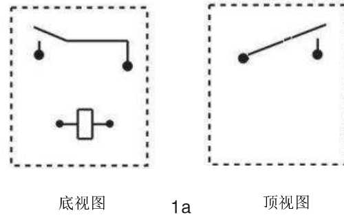
接线图 WIRING DIAGRAM
