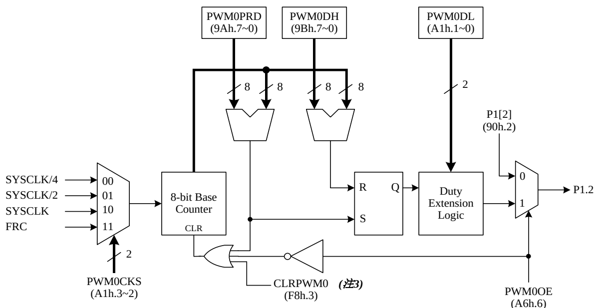
PWM0 结构
