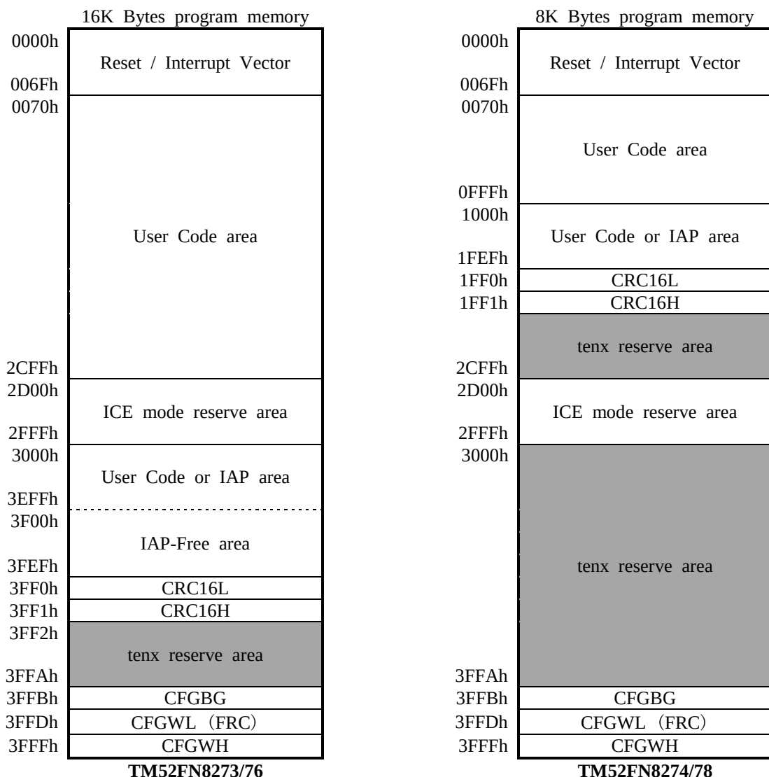
TM52FN8273/76
