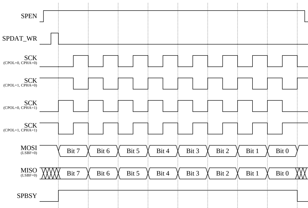
主模式时序
