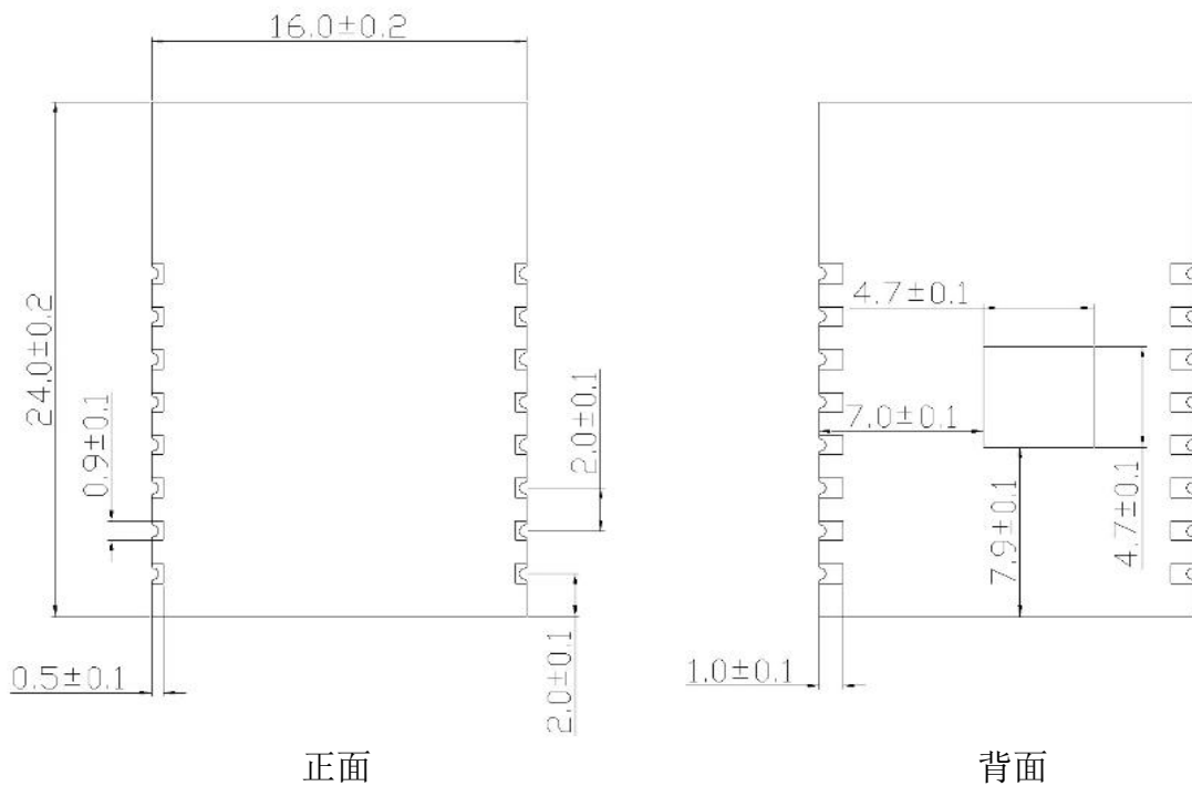
图 4 尺寸图
