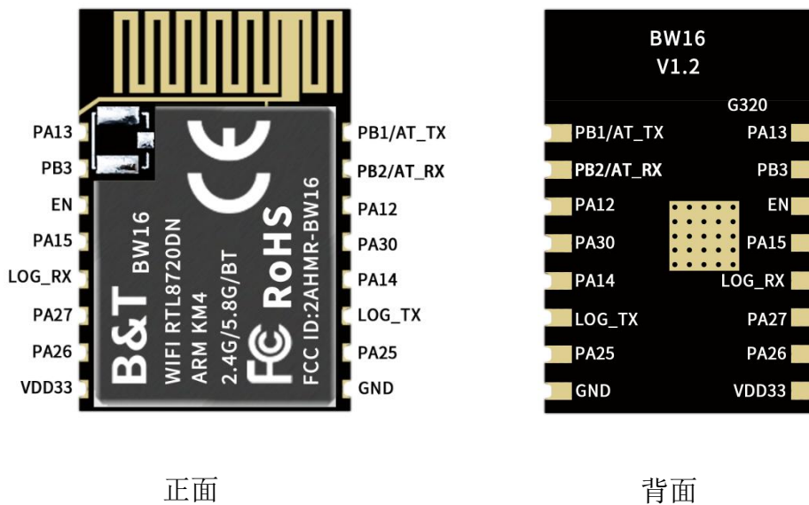
图 6 管脚示意图
