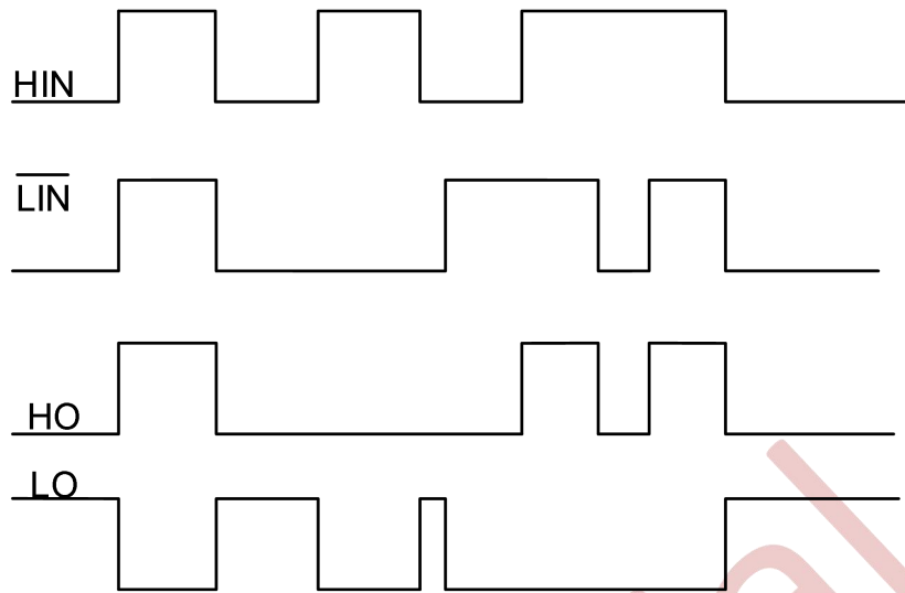
图 9-1 G2022Q 输入输出时序波形
