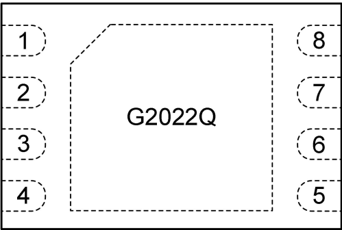
图 7-1 8-脚 DFN 顶视图
