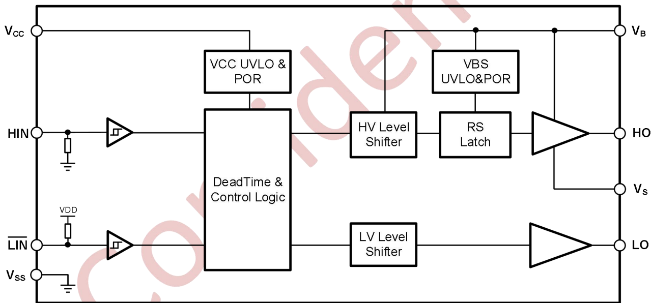
图 10-1 G2022Q 功能框图
