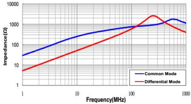
XRACM4520F-701
