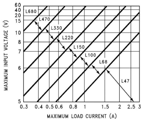
LM2576-3.3
