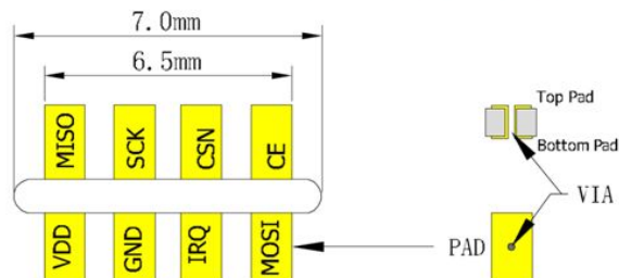
PCB 主板开槽尺寸示意
