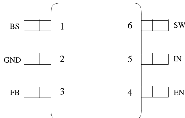
SOT23-6 (SDA616)
