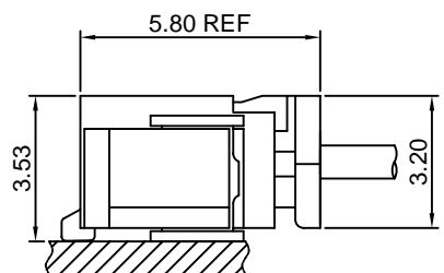
SMT TYPE
