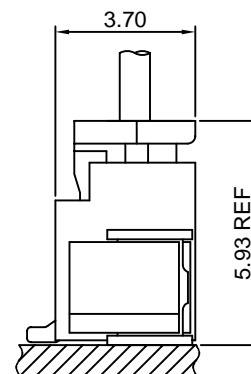
SMT TYPE
