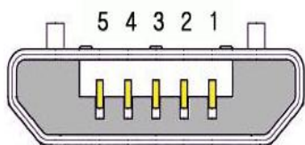
micro-USB 公头
