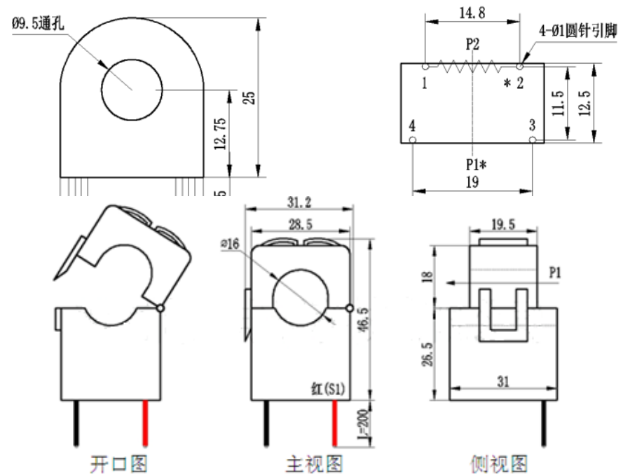
100A 开口式电流互感器外形尺寸图
