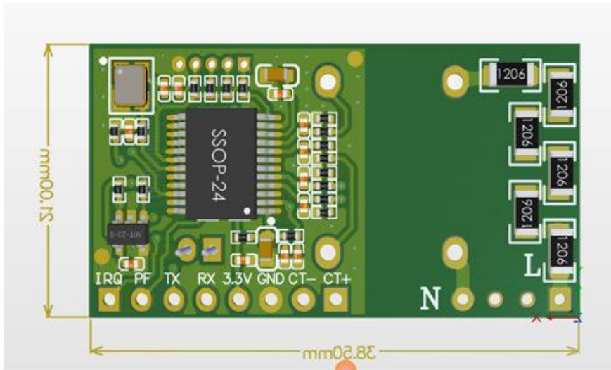
图示 外形尺寸图 (单位:mm)
