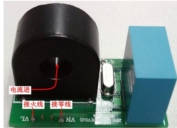
接线示意图
