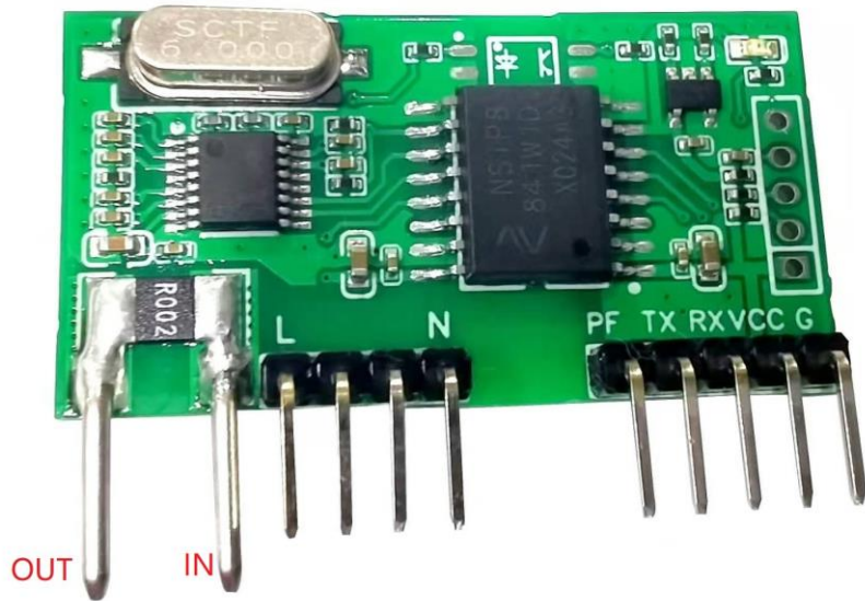
图 2.1 外形图
