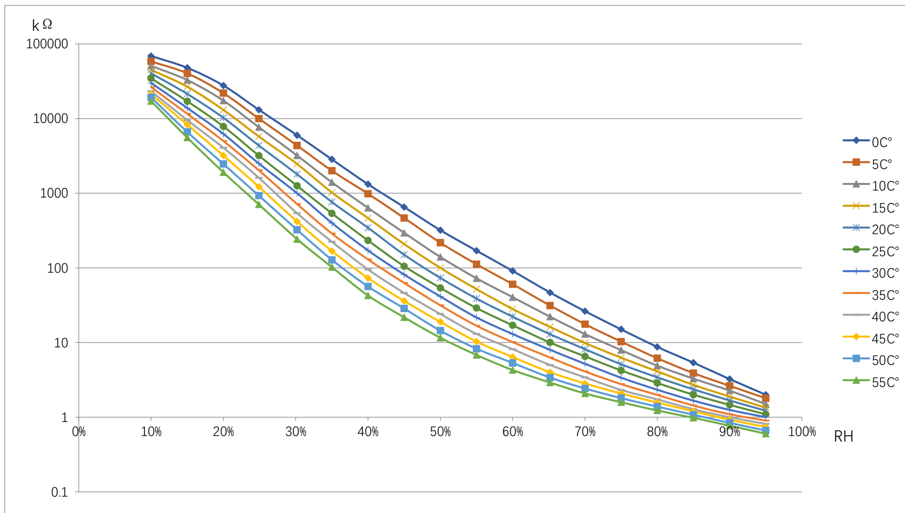
附件 2: HGS10 温湿度特性曲线
