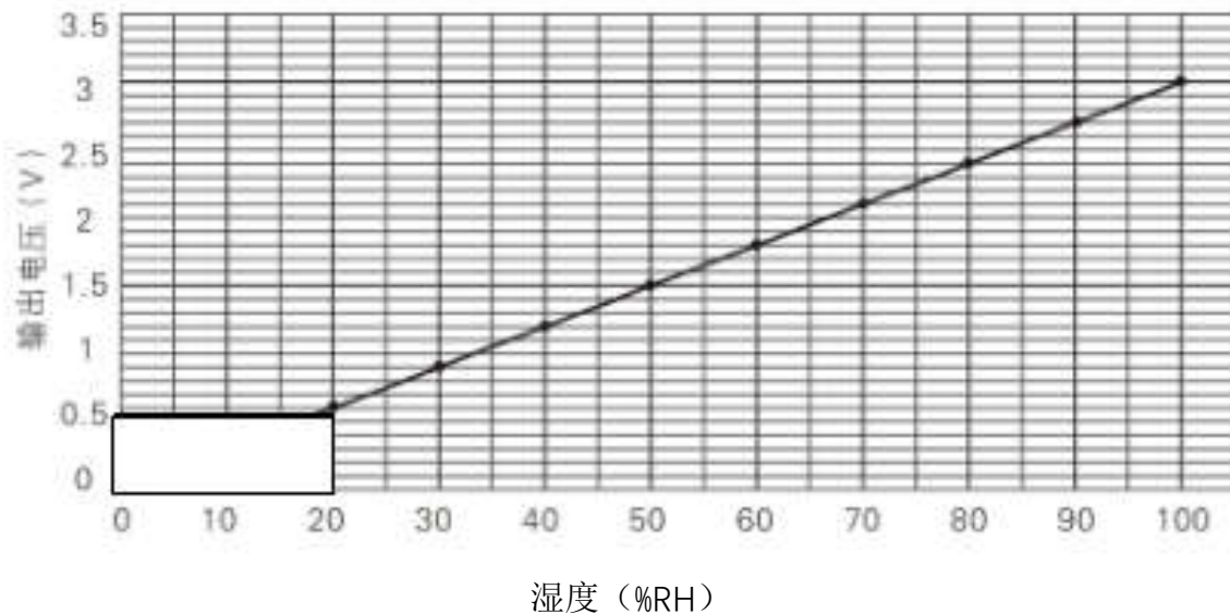
电压输出与湿度的线性曲线图
