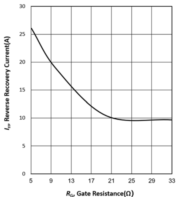
图 8 二极管反向恢复峰值电流与栅电阻的关系 ( T_{vj}=25^{\circ}\text{C} , V_{CE}=600\text{V} , I_F=50\text{A} )
