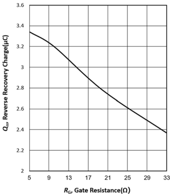
图 7 二极管反向恢复电荷与栅电阻的关系 ( T_{vj}=25^{\circ}\text{C} , V_{CE}=600\text{V} , I_F=50\text{A} )
