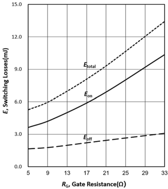
图 5 IGBT 开关损耗与栅极电阻的关系 (感性负载, T_{vj}=25^{\circ}\text{C} , V_{CE}=600\text{V} , V_{GE}=0/15\text{V} , I_C=50\text{A} )
