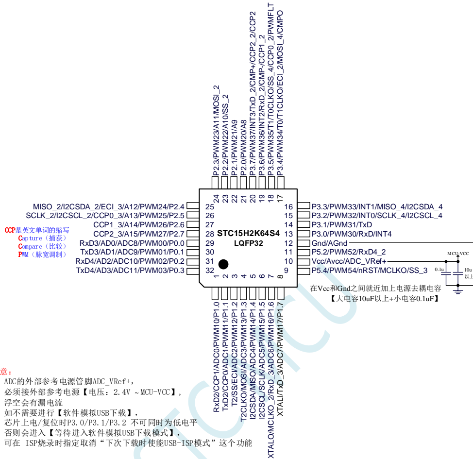
STC15H2K64S4-LQFP32 最小系统 示意图
