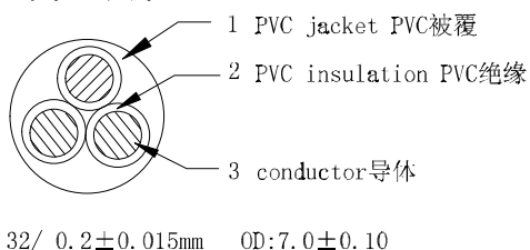
线材截面图:
