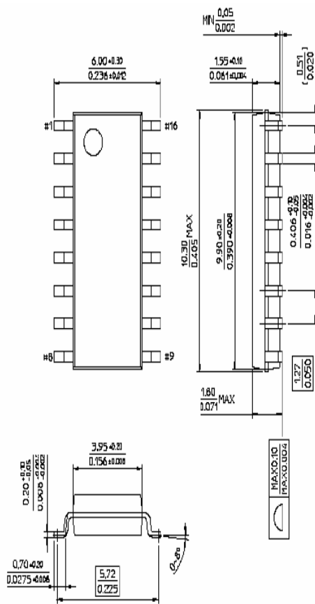
SOP16 外形尺寸图
