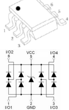
SOT-23-6L
