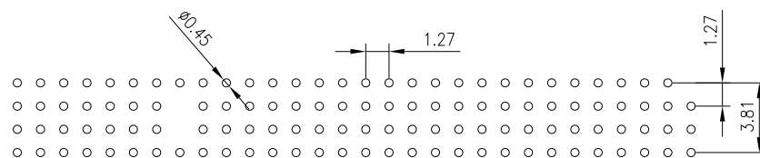
P.C.B LAYOUT
