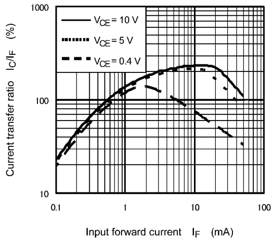
Fig. 11.11 I_C/I_F - I_F
