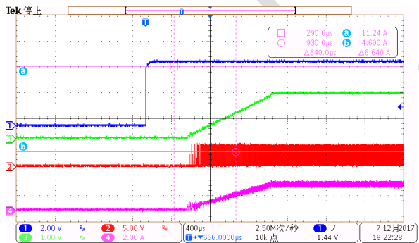
EN on, Iout= 2A
