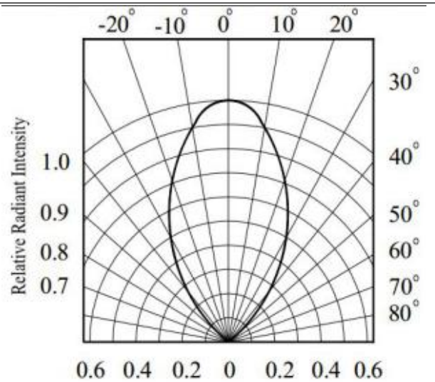
发射角度图
