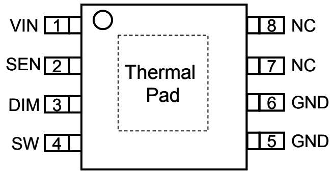
MBI6655GD (正面)
